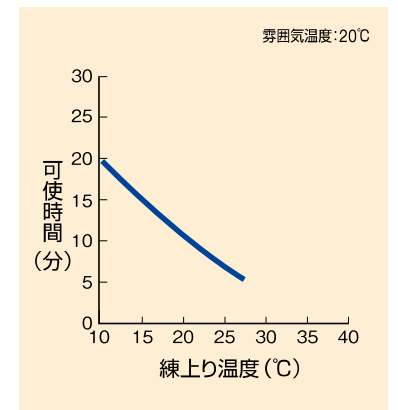
練上り温度と可使時間の関係
